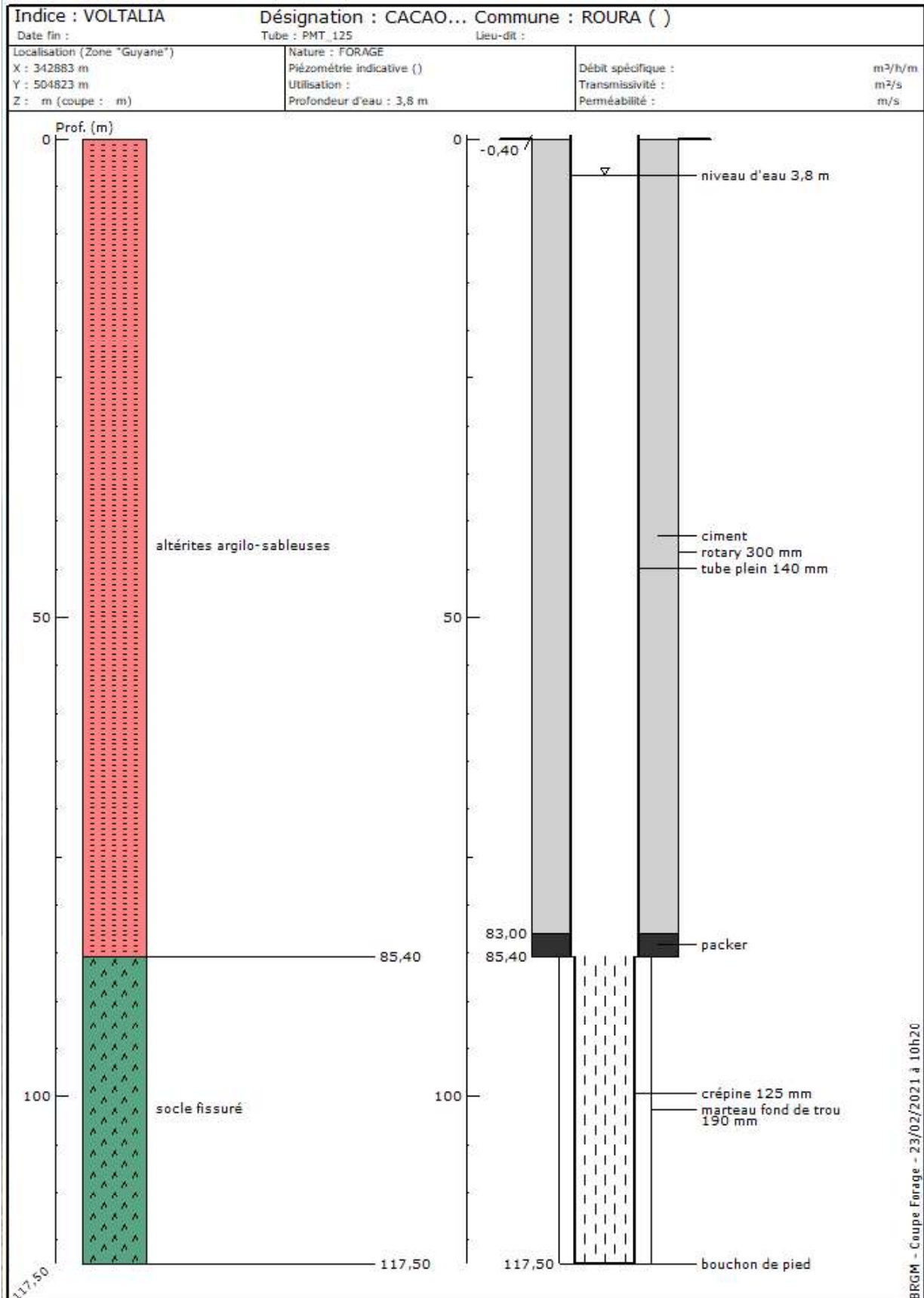
Figure 3: Coupe géologique et technique du forage de la centrale de Voltalia (BRGM)
